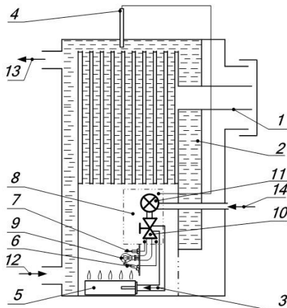
Рисунок 4.3 Функциональная схема котла с автоматикой безопасности и регулирования EUROFIT 630, TGV-306, TGV-307.
