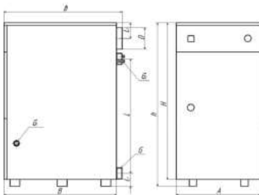
Рисунок 4.1 Габаритные и присоединительные размеры трубного котла.
